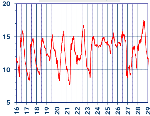
PRESSIONE, mbar
